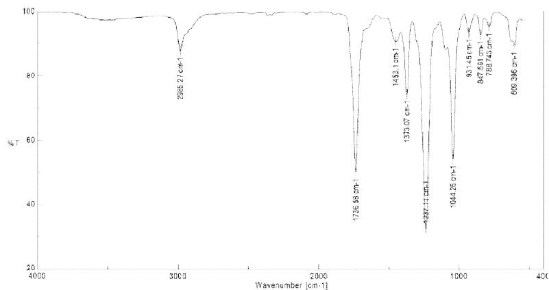
Fig. 3. FTIR spectrum
